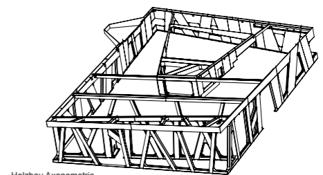
Holzbau Axonometrie
