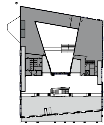
Galeriegeschoss M. 1: 500
